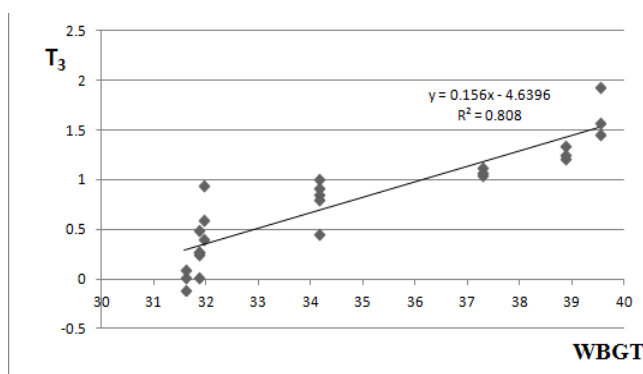
شکل ۱- رابطه تغییرات T3 با دمای هوا و WBGT در افراد مورد مطالعه
