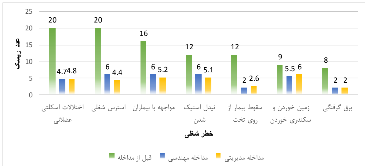
نمودار ۱. مقایسه عدد ریسک خطرات شغلی در وظیفه‌ی پرستار تربیاز قبل و بعد از اجرای کنترل‌های مدیریتی و مهندسی
