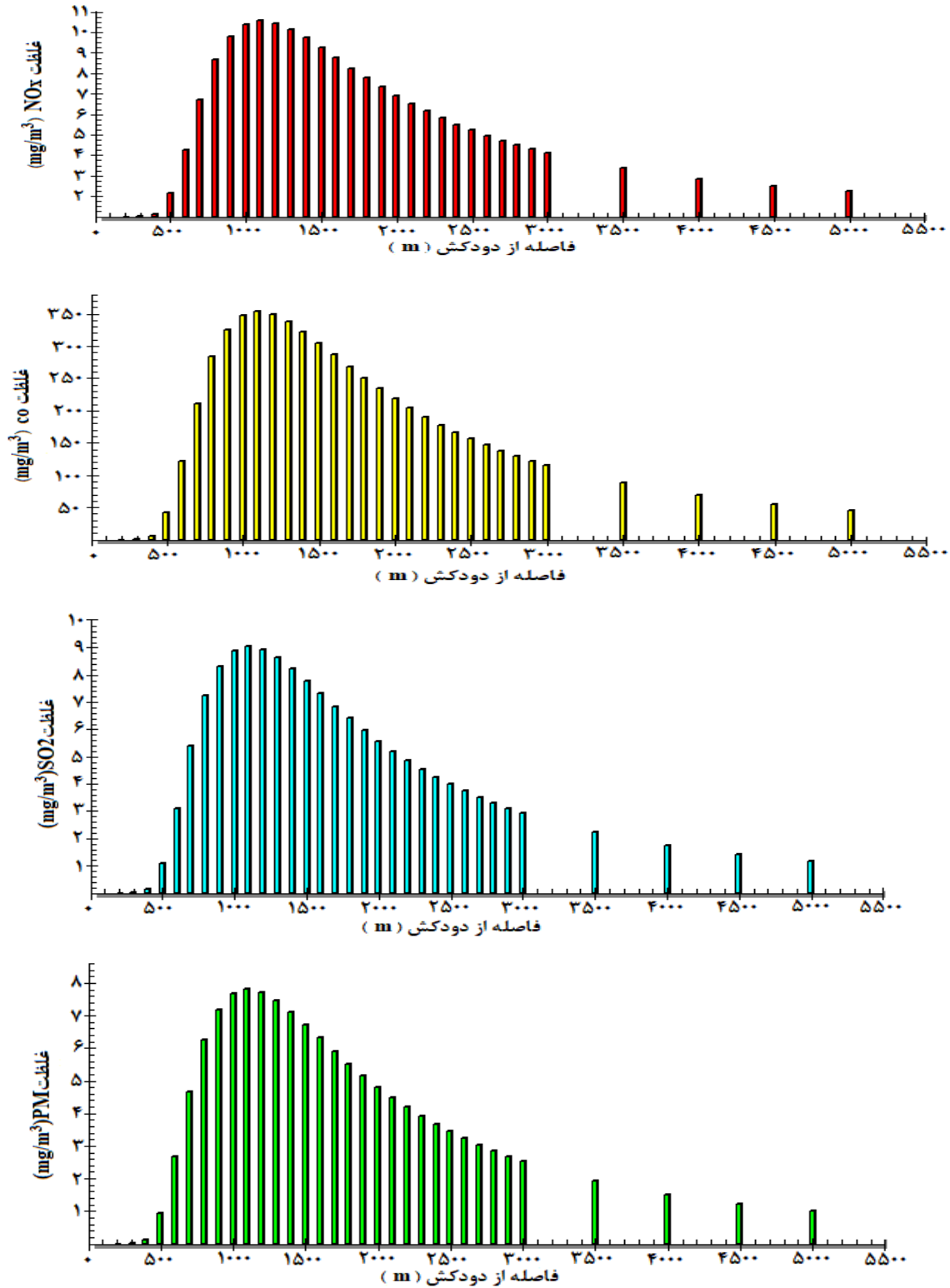
شکل ۴. بیشترین غلظت NO_x (قرمز رنگ)، CO (زرد رنگ)، SO_2 (آبی رنگ) و PM (سبز رنگ) ناشی از سوخت مازوت، در پایین دست جهت باد نسبت به فاصله از دودکش کارخانه سیمان سبزوار در شرایط جوی ناپایدار و سرعت باد ۵ متر بر ثانیه
