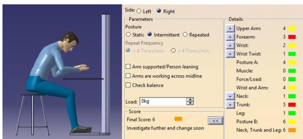
شکل ۳. تحلیل وضعیت سمت راست بدن در وضعیت اولیه به روش RULA در هنگام جوشکاری
