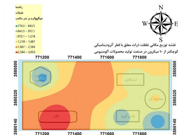
شکل ۱۰. توزیع مکانی تراکم جرمی PM_{10} در صنعت تولید محصولات آلومینیومی
