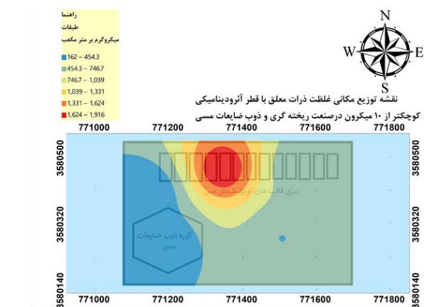
شکل ۱۲. توزیع مکانی تراکم جرمی PM_{10} در صنعت ریخته گری و ذوب ضایعات مسی
