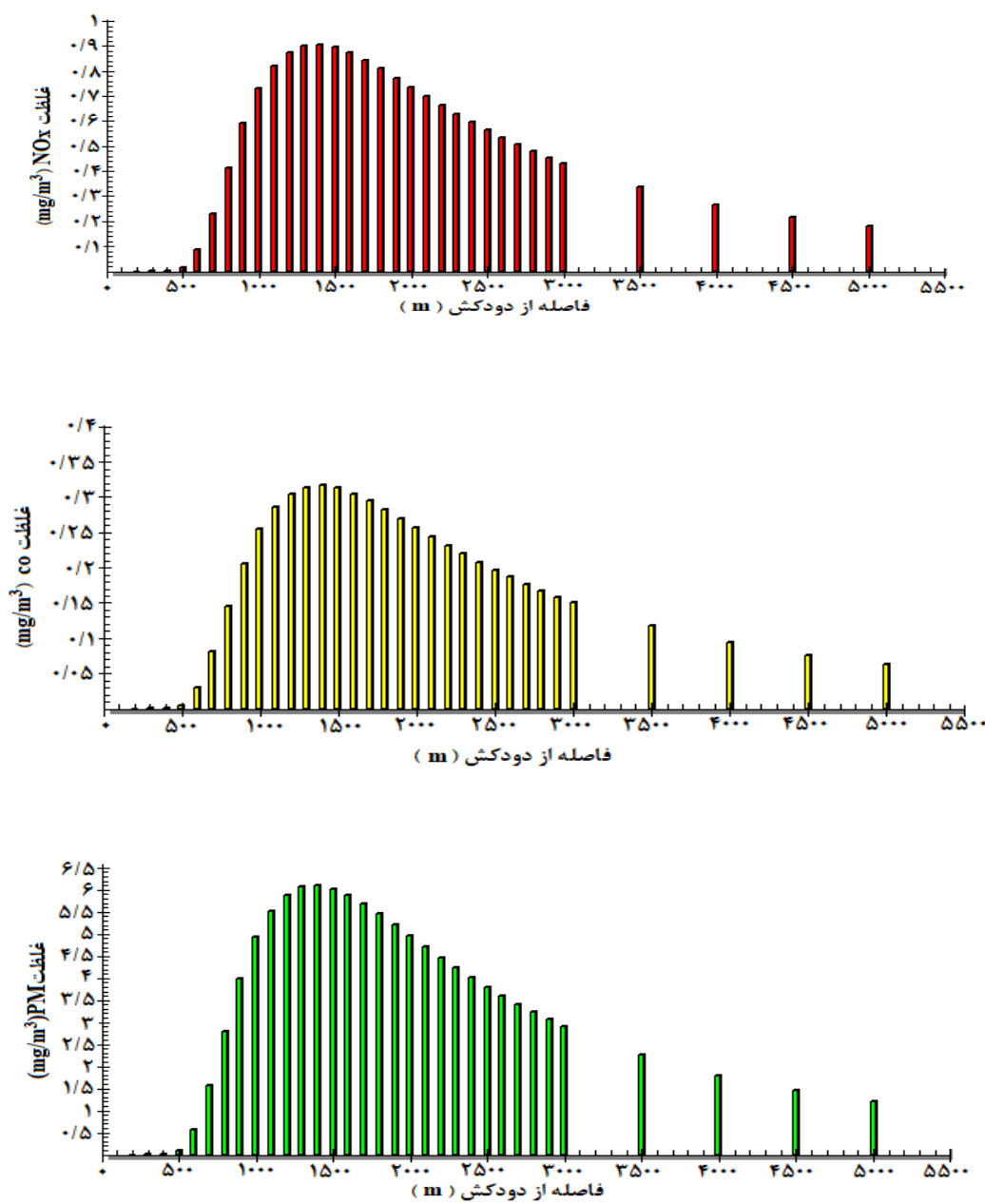
شکل ۳. بیشترین غلظت \text{NO}_x (قرمز رنگ)، CO (زرد رنگ) و PM (سبز رنگ) ناشی از سوخت گاز، در پایین دست جهت باد نسبت به فاصله از دودکش کارخانه سیمان سبزوار در شرایط جوی ناپایدار و سرعت باد ۵ متر بر ثانیه
