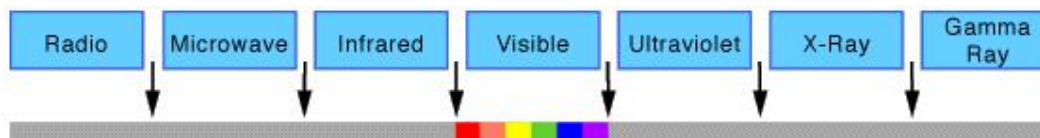
شکل ۱: طیف الکترومغناطیس
